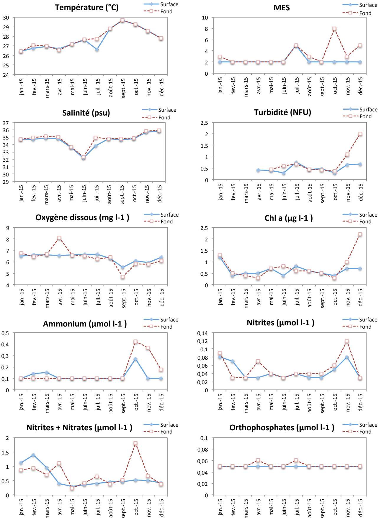
Figure 9 : Résultats mensuels de chaque paramètre pour la station Gros Ilet (204).
