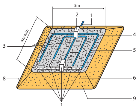
Vue de dessus du tertre d'infiltration non drainé ( K > 200 \text{ mm/h} )
