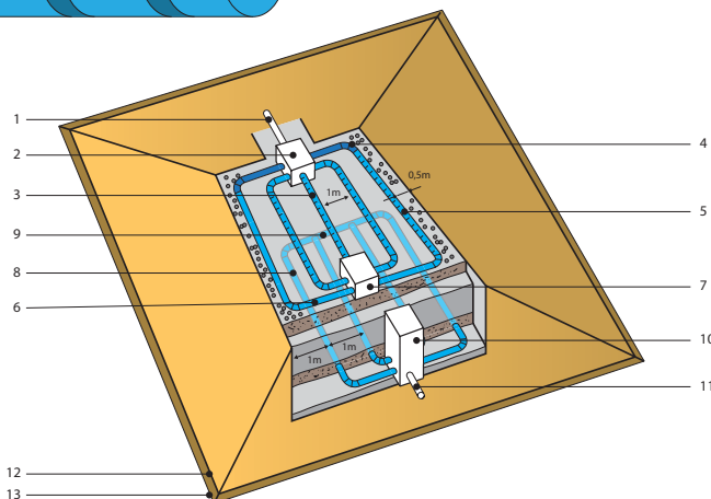
Vue de dessus du tertre d'infiltration drainé ( K < 15 \text{ mm/h} )
