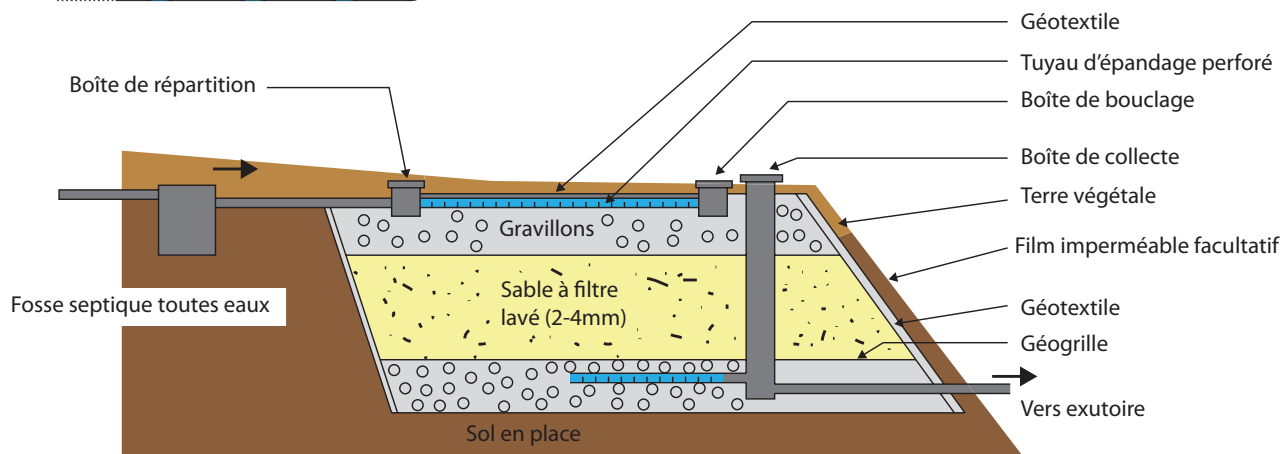
Coupe longitudinale
