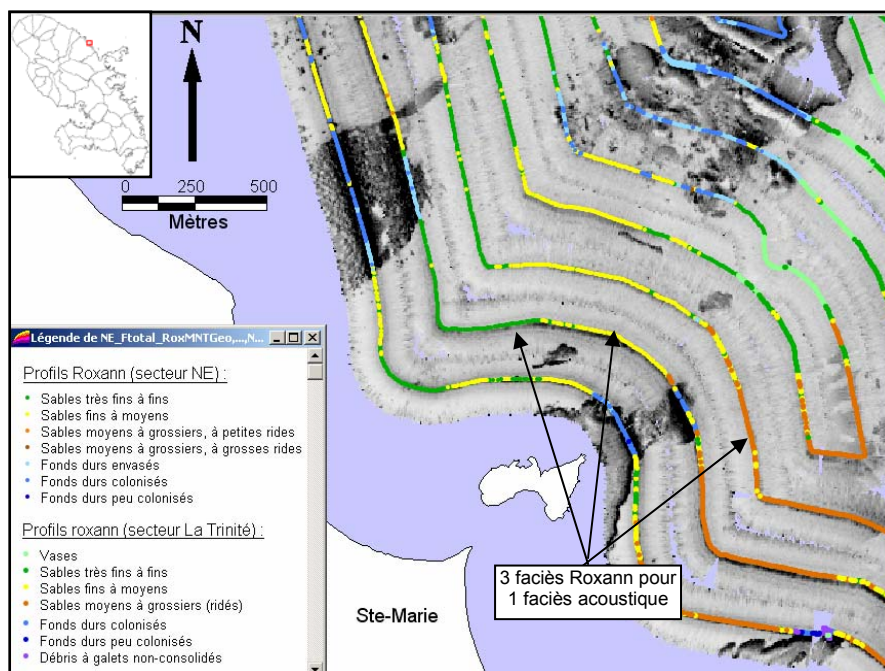
Figure 23 – Exemple de discrimination plus importante des faciès meubles par le système Roxann dans certain secteurs (reportée sur imagerie Geoswath)
