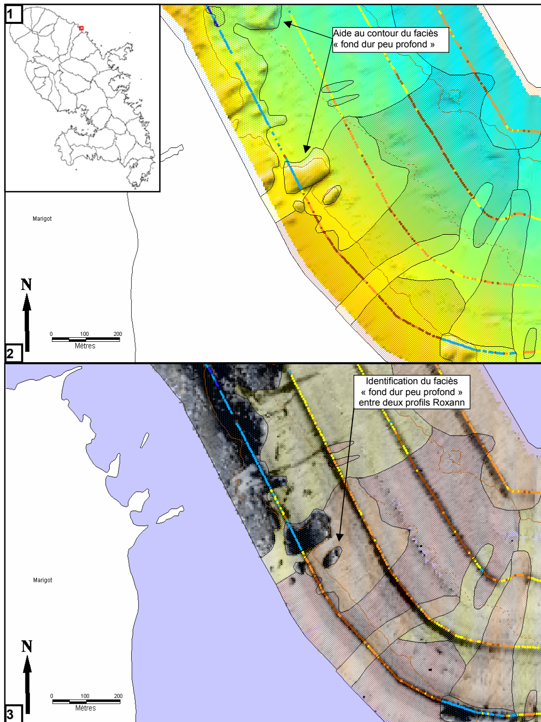
Figure 20 - Exemple d'aide à la numérisation des limites de faciès par la bathymétrie et l'imagerie acoustique (1 : localisation de la zone ; 2 : apport de la bathymétrie ; 3 : apport de l'imagerie acoustique)
