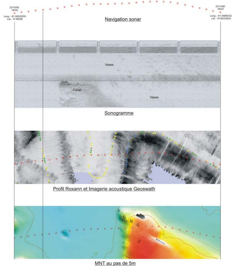
Figure 25 – Comparaison des données d'imagerie acoustique (sonar latéral en haut, imagerie Geoswath au milieu) et morphologie détaillée (en bas). Exemples de la baie de Fort de France (à gauche) et du secteur NE (à droite).
