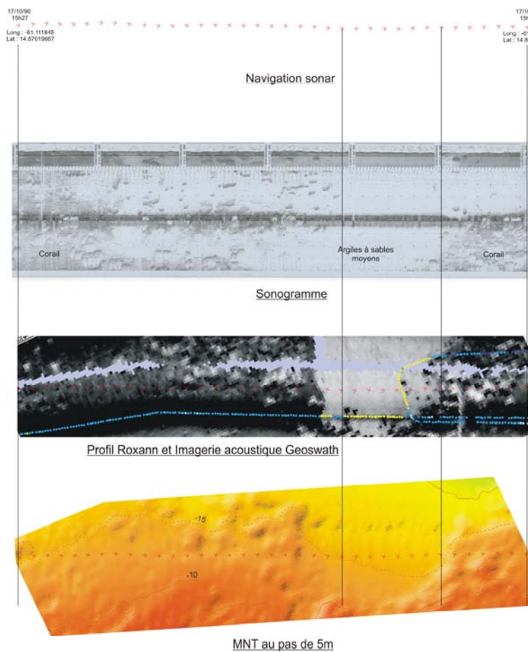
Figure 25 – Comparaison des données d'imagerie acoustique (sonar latéral en haut, imagerie Geoswath au milieu) et morphologie détaillée (en bas). Exemples de la baie de Fort de France (à gauche) et du secteur NE (à droite).
