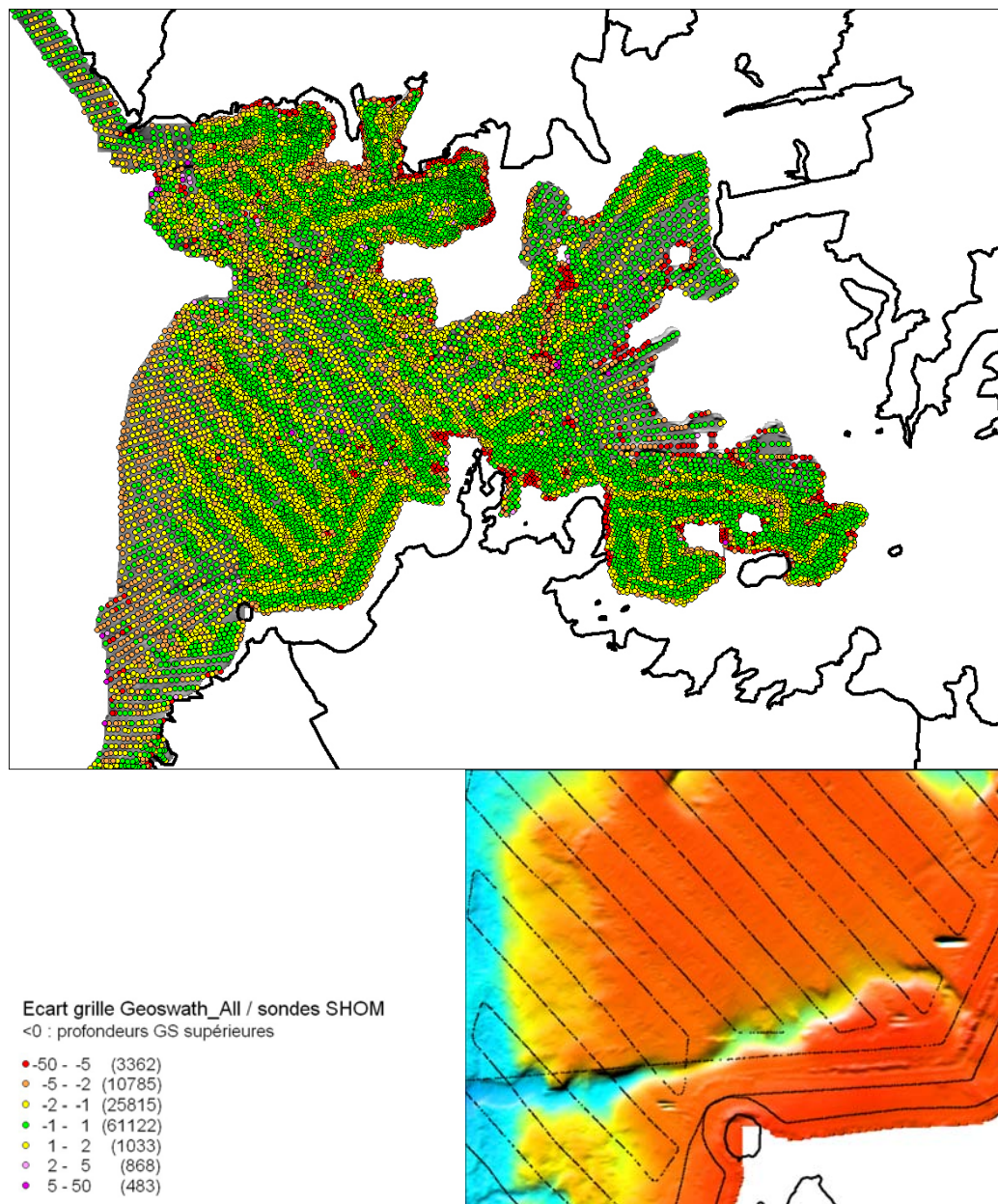
Figure 10 –Ecart entre les valeurs de bathymétrie du levé Geoswath et les sondes du SHOM dans la baie de Fort de France ; la distribution des écarts (par classes de valeurs) suit la localisation des profils (écarts > 1m en jaune)
