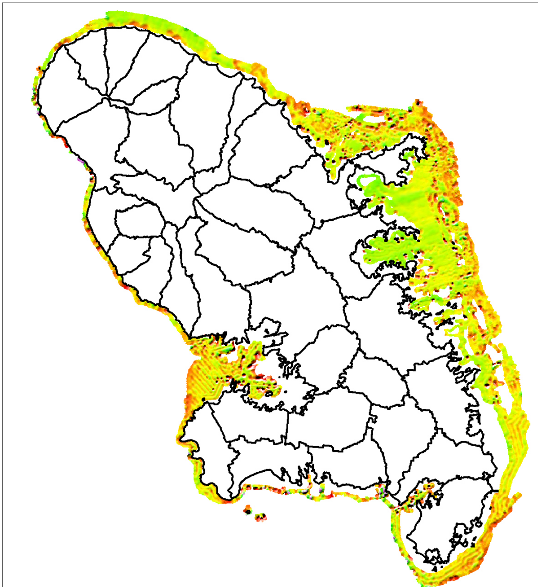
Figure 11 - Vue synthétique (modèle maillé) sur l'ensemble du domaine côtier des écarts entre valeurs de bathymétrie du levé Geoswath et sondes du SHOM (en rouge : écarts > 5m, en vert écarts < 1 m).
