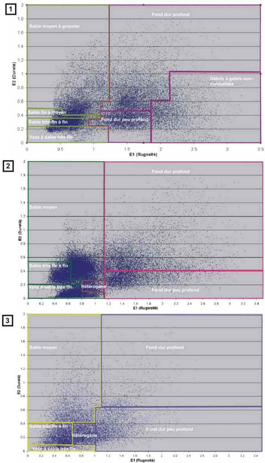
Figure 18 –Calibration des faciès Roxann des autres zones : 1 : La Trinité ; 2 : baies du Galion et du Robert ; 3 : baie de Fort de France.
