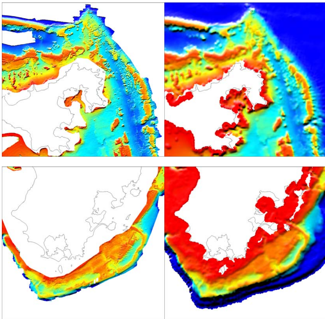
Figure 9- Exemples de morphologies détaillées révélées par le nouveau levé côtier (à gauche) et comparaison avec un MNT au pas de 25 mètres calculé à partir des sondes du SHOM (à droite)
