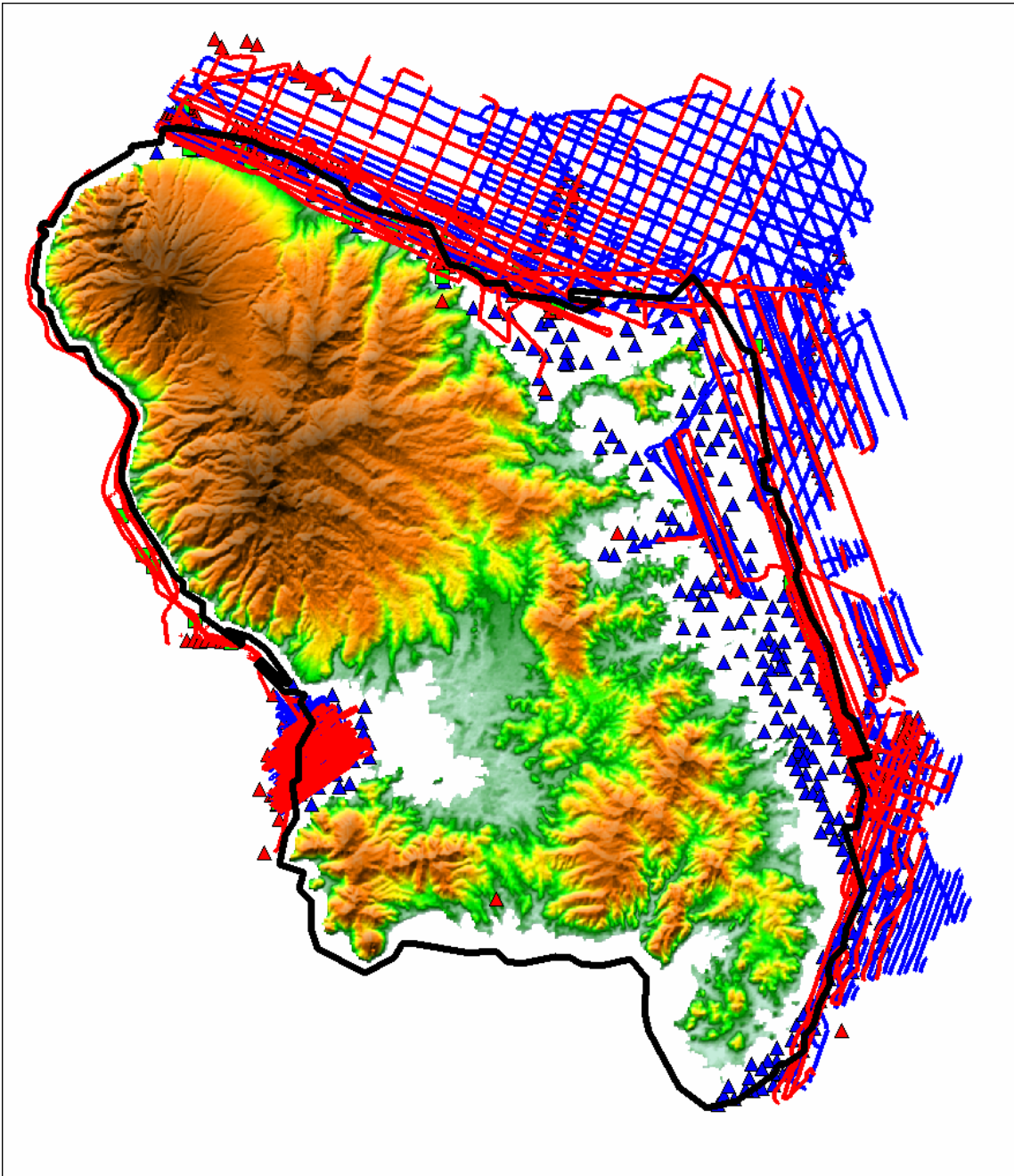
Figure 13 – Localisation des données antérieures recueillies par Ifremer et l'Université de Bordeaux : profils de sonar latéral et prélèvements de sédiments.
