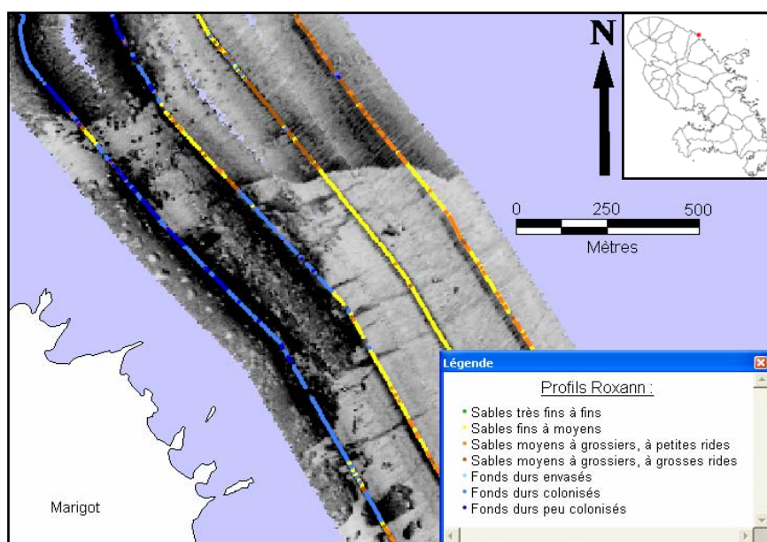
Figure 22 - Exemple dans le secteur NE de discrimination plus importantes des fonds durs du système Roxann sur le Geoswath
