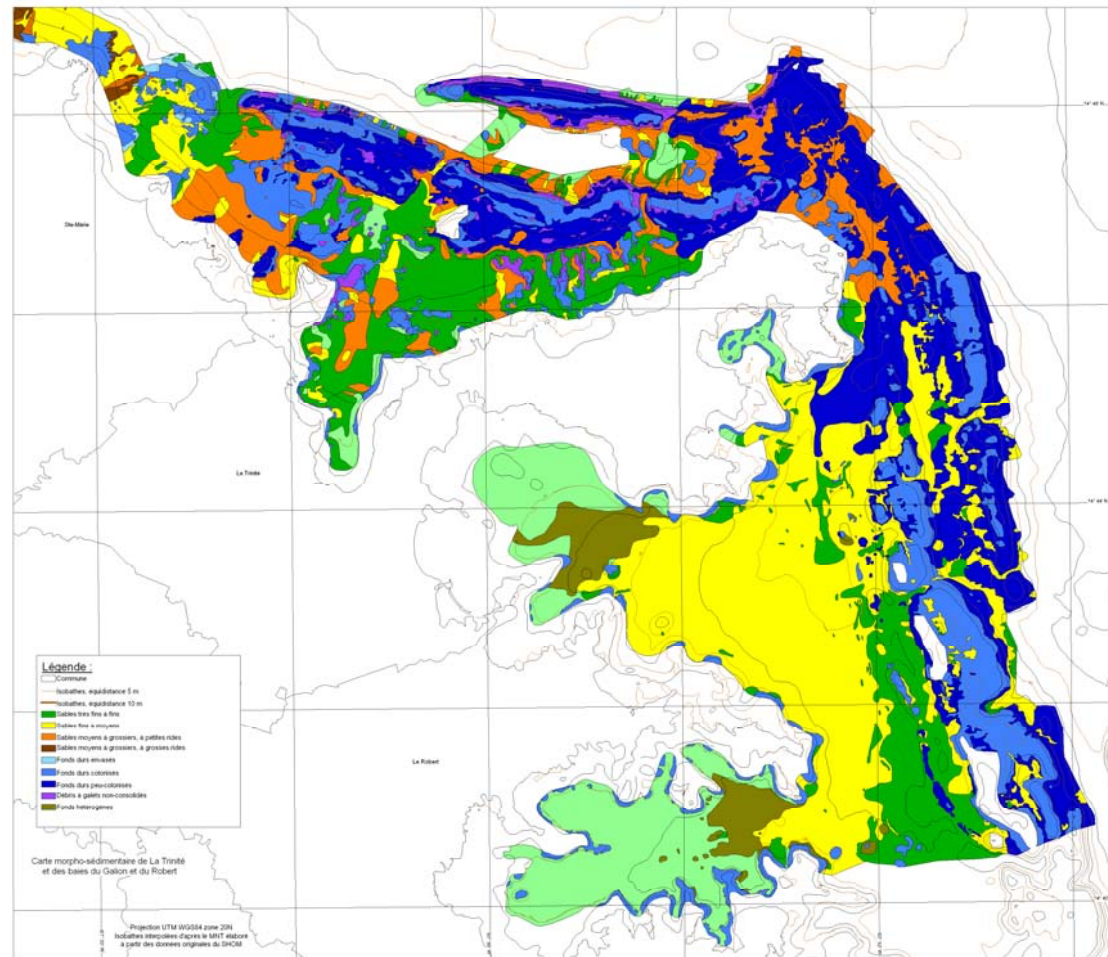
Figure 29 – Carte sédimentologique de la Trinité au havre du Robert
