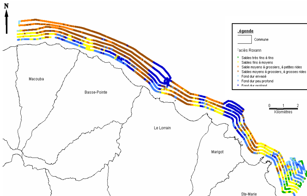
Figure 17 – Exemple de distribution des faciès Roxann le long de la côte nord : la classification des faciès à partir des données Roxann met en évidence les principaux domaines sédimentaires
