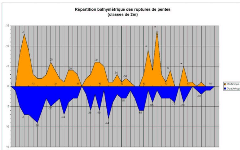
Figure 5 – Distribution des ruptures de pentes sur les plates-formes de la Martinique et de la Guadeloupe (Duclos, 2007)
