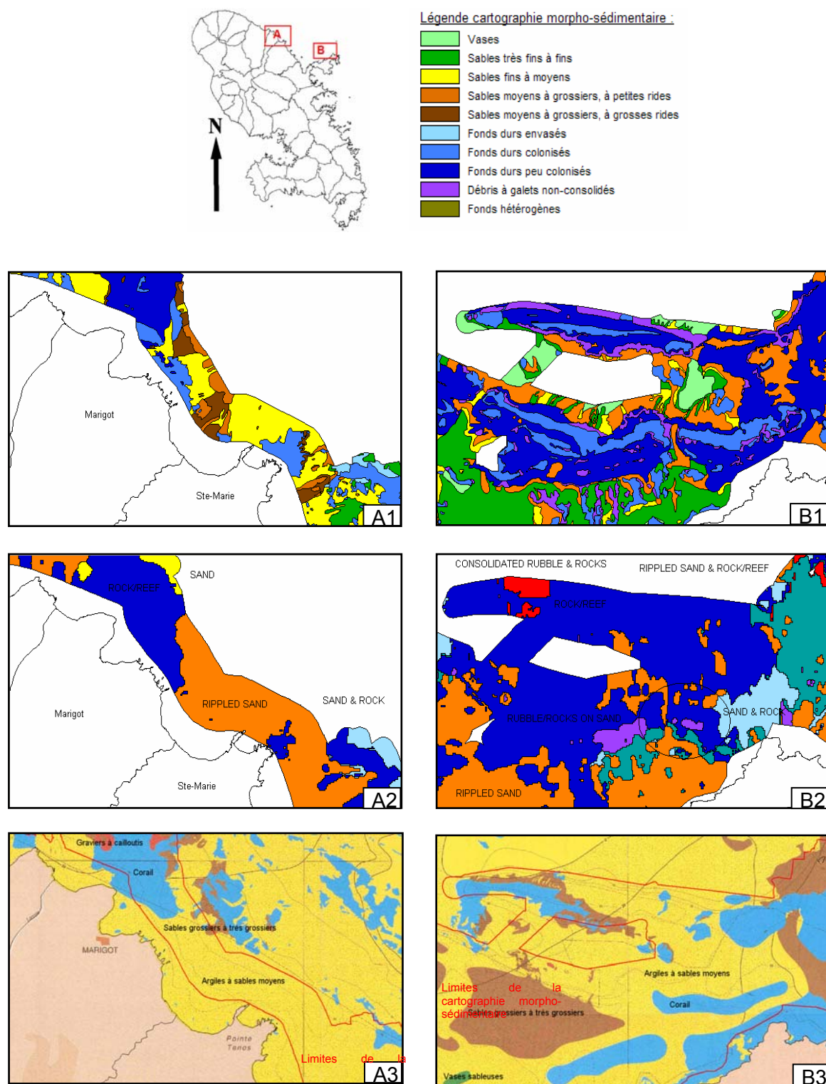
Figure 31 – Comparaison des 3 types de cartographie réalisées dans dans deux secteurs (A et B) de la zone côtière nord-est : 1: cette étude, 2: Envision 2007 ; 3: Ifremer : 2000
