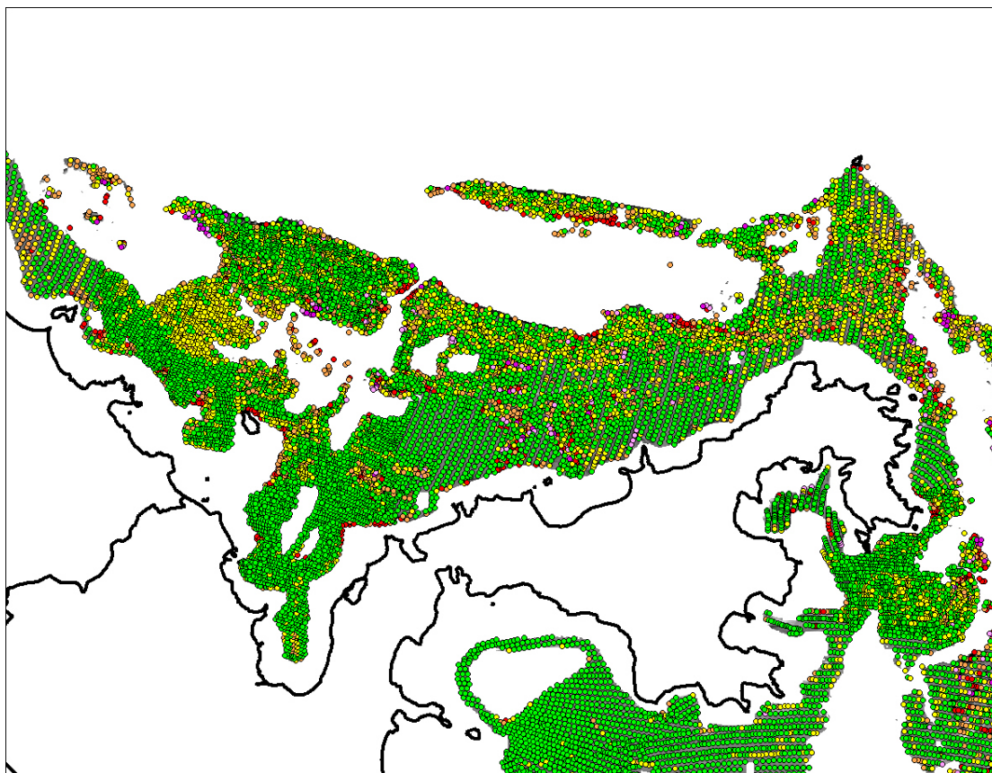
Figure 12 – Ecart entre les valeurs de bathymétrie du levé Geoswath et les sondes du SHOM Code des couleurs : voir Figure 10
