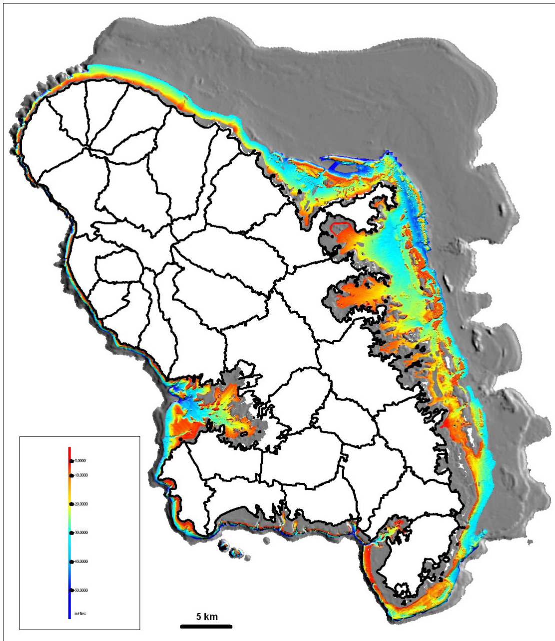
Figure 7- MNT à la maille de 5mètres de la zone côtière de la Martinique issu des levés Envision (données août 2007) (en couleur) superposé au MNT de la plate-forme calculé à partir des données du SHOM (en ombré).
