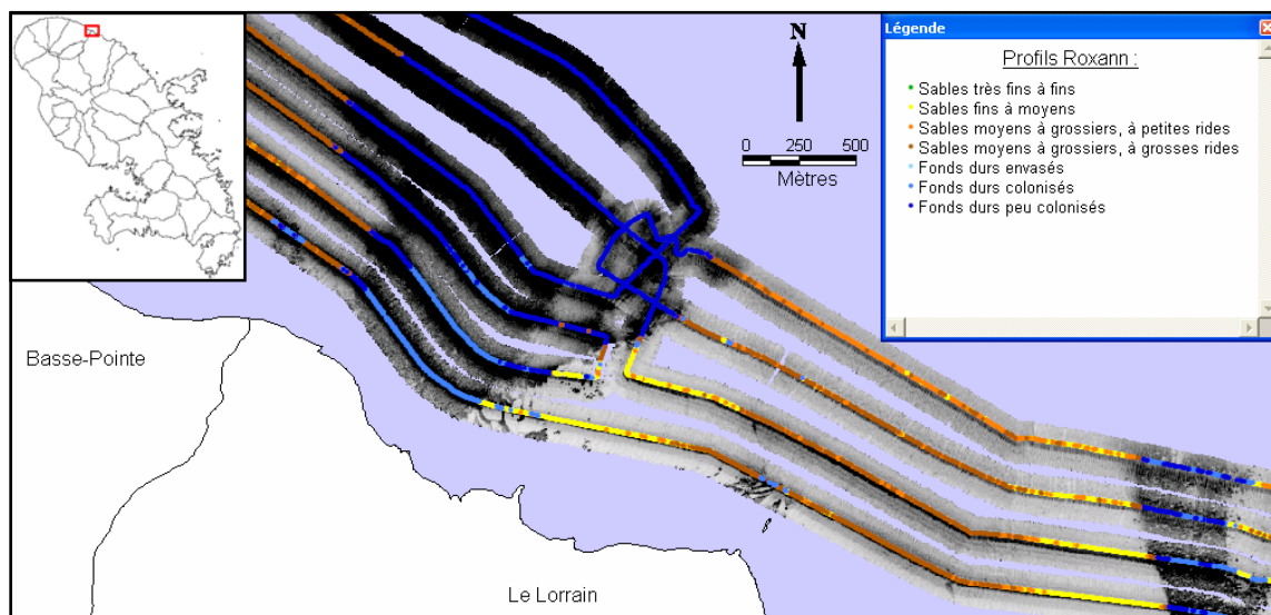
Figure 21 - : Exemple de cohérence entre les données Roxann et Geoswath dans le secteur N. Note : sur les figures 20 à 24, les « faciès Roxann » sont représentés par les séries de points de couleur le long des profils sur les images de bathymétrie ou de réflectivité Geoswath.
