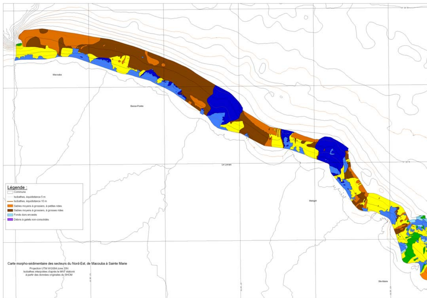
Figure 28 – Carte -sédimentologique du secteur Nord-Est
