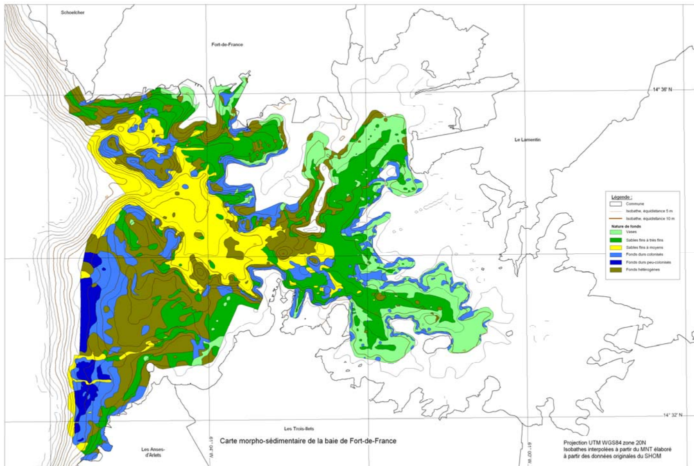
Figure 27 – Carte sédimentologique de la baie de Fort de France
