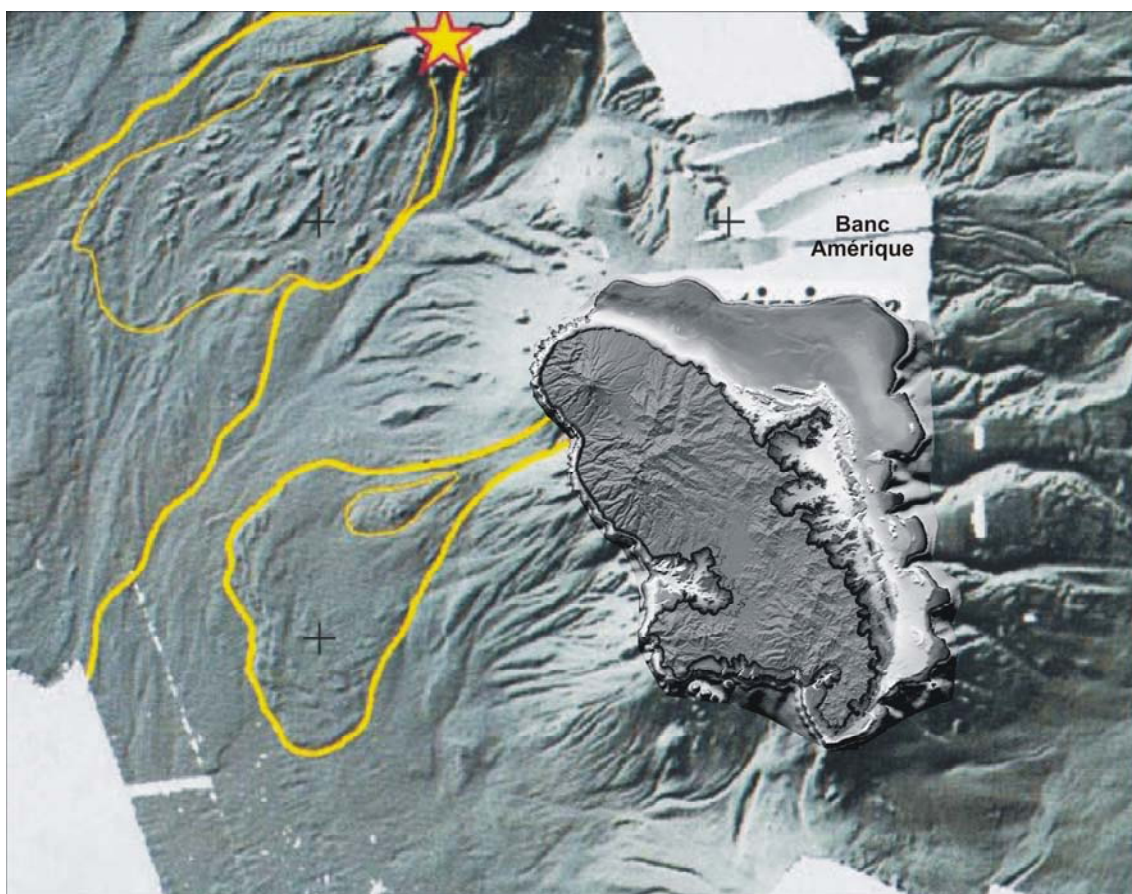
Figure 6 – Cadre morphologique régional de la Martinique : Image des MNT terre IGN et plate-forme (0-100m) d'après les données du SHOM replacé sur l'image du MNT ombré des pentes
