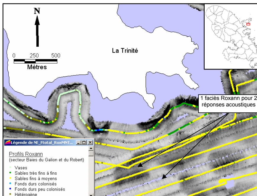
Figure 24 – Exemple de discrimination plus importante des faciès meubles par l'imagerie acoustique Geoswath
