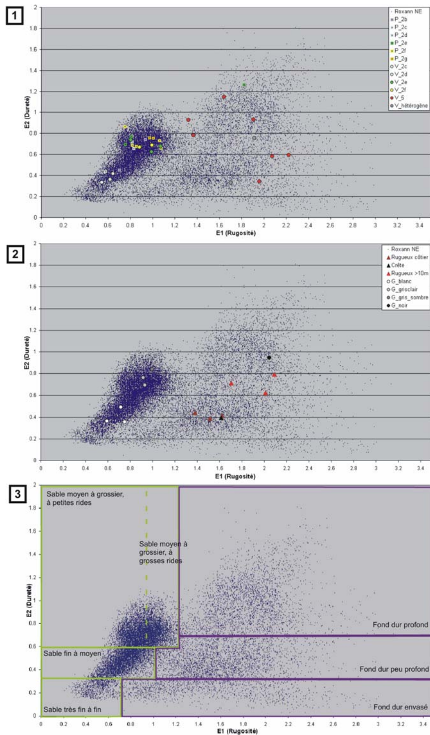
Figure 16- Calibration des données Roxann et création de « boîtes » ou secteurs de faciès. 1 : calibration avec données directes ; 2 : calibration avec données indirectes, G faciès de réflectivité Geoswath ; 3 : délimitation des faciès
