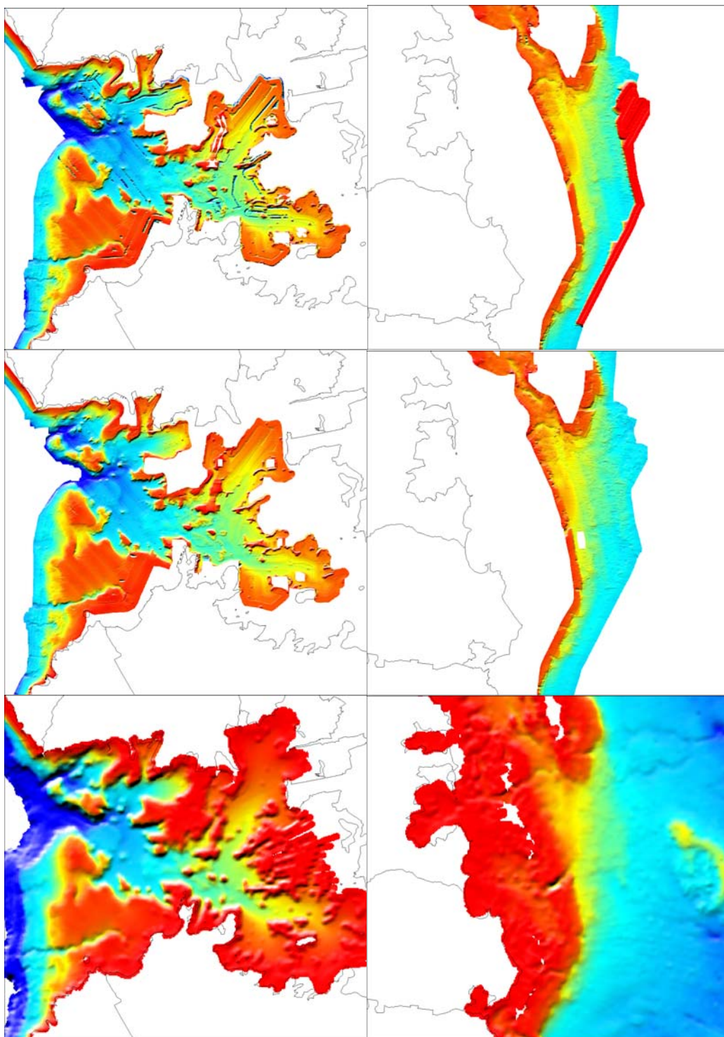
Figure 8 - Comparaison des MNT de la baie de Fort de France( à gauche) et du secteur SE (à droite) ; de haut en bas : MNT 5m provisoires Envision, définitifs, MNT25m (établi à partir des données SHOM).
