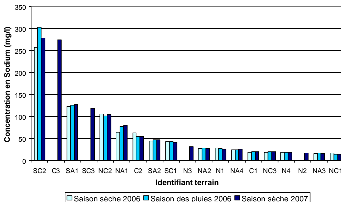
Illustration : Histogramme des concentrations en sodium mesurées en saison sèche 2007
