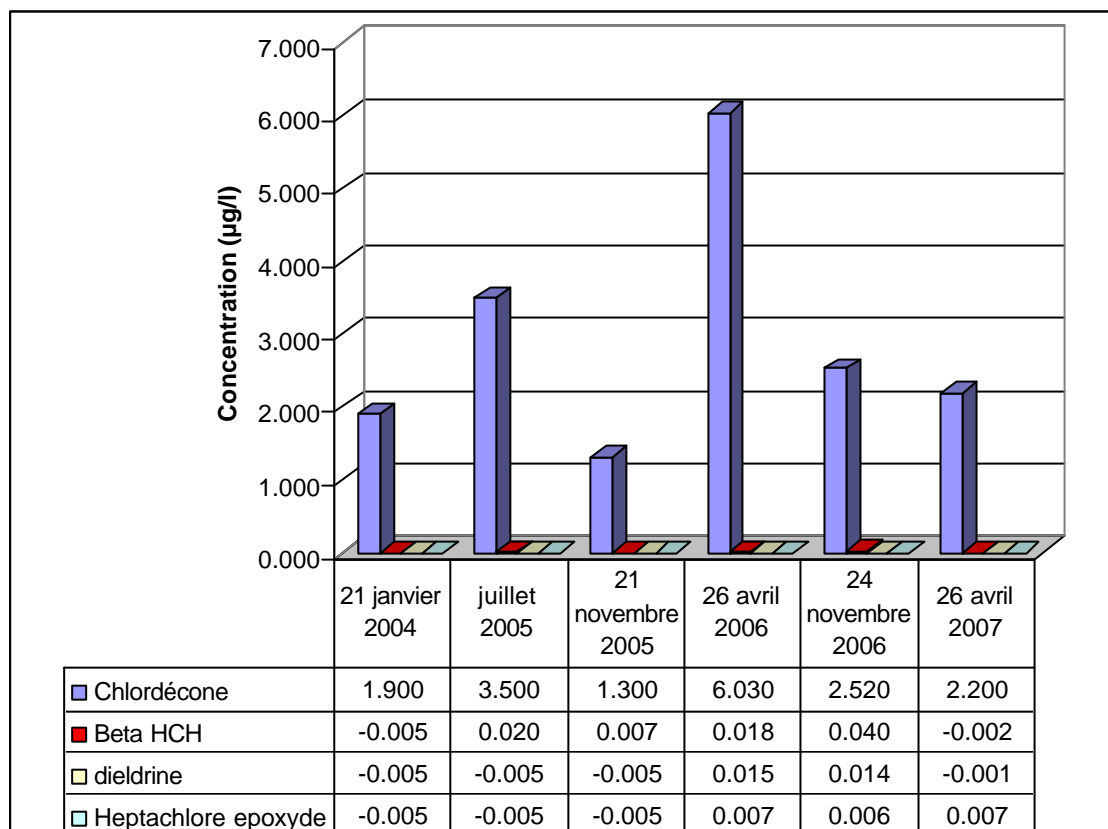
Illustration 37 : Produits phytosanitaires détectés sur le site de Trinité – Source Morne Figure
