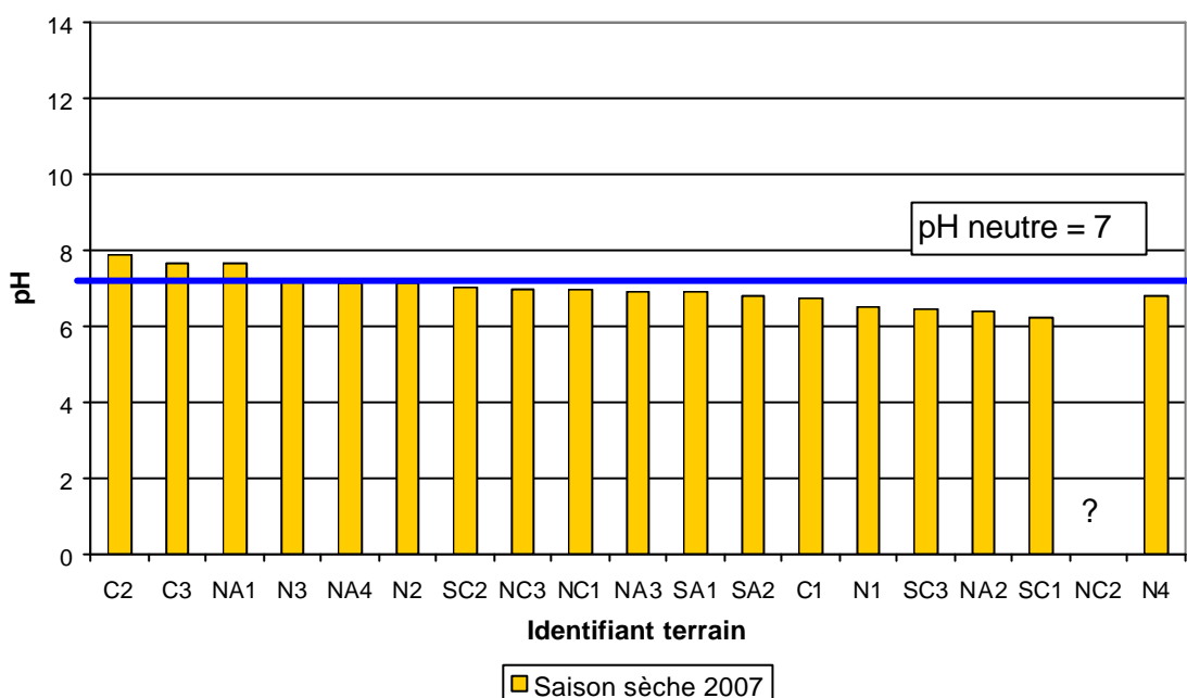
Illustration 8 : pH mesurés in situ lors de la campagne de saison sèche 2007
