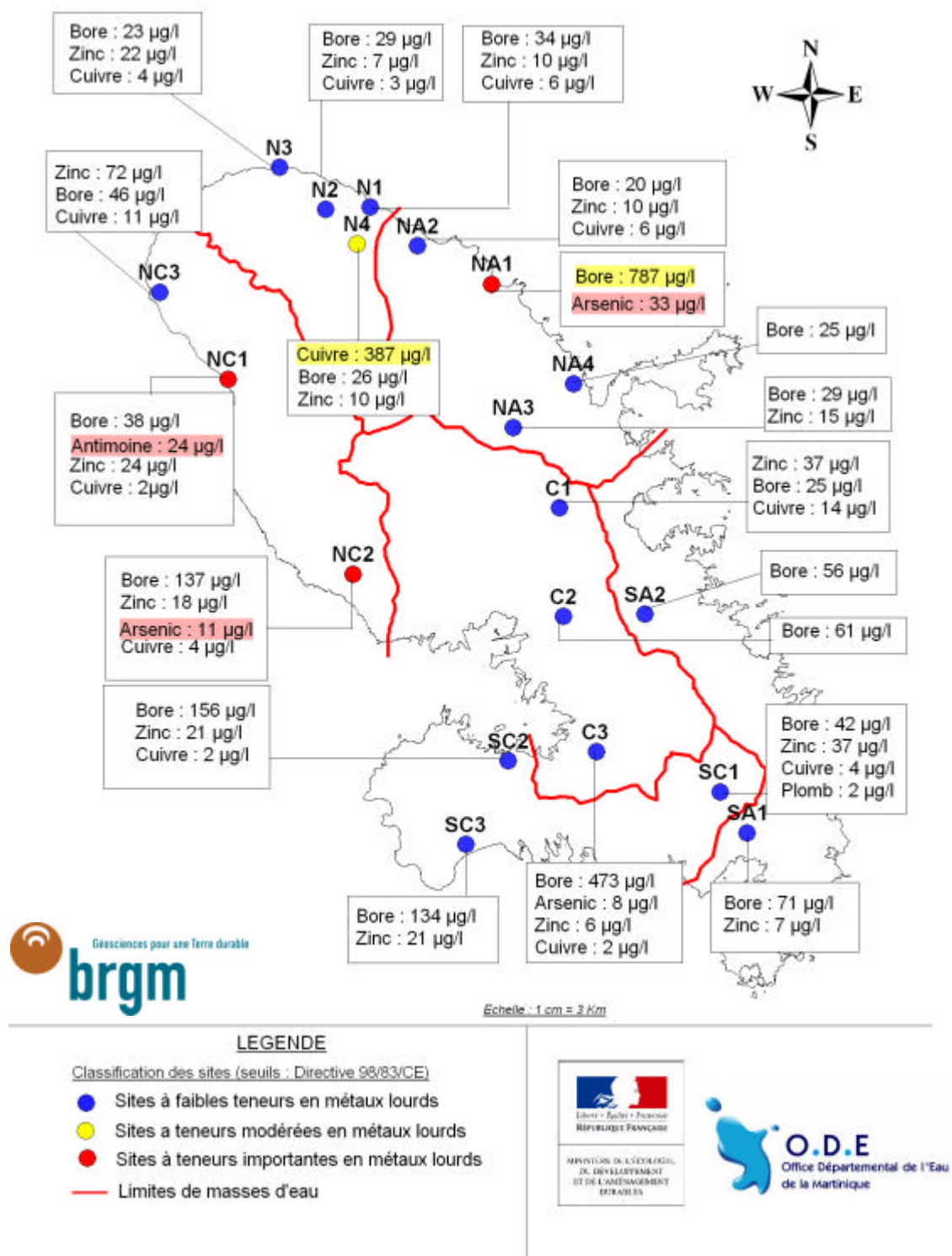
Illustration 30 : Carte de synthèse des métaux lourds retrouvés dans les eaux souterraines
