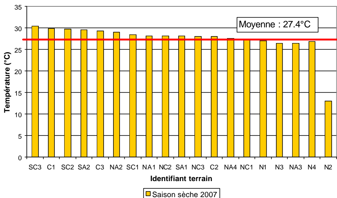
Illustration 6 : Températures relevées in situ lors de la campagne de saison sèche 2007
