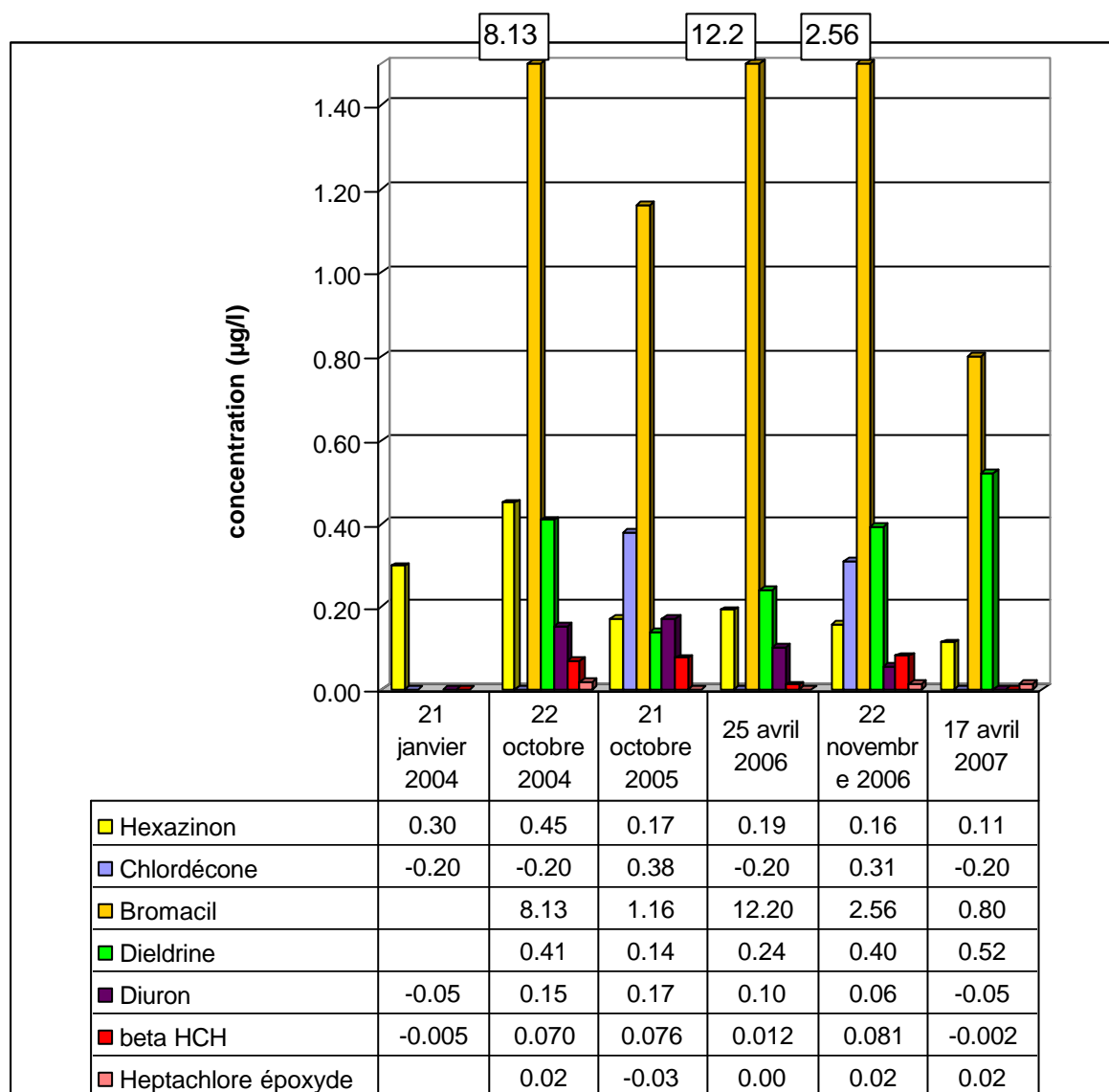
Illustration 40 : Produits phytosanitaires détectés sur le site de Basse Pointe – Rivière Falaise
