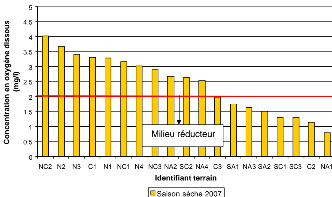
Illustration 9 : Teneurs en oxygène dissous mesurées in situ lors de la campagne de saison sèche 2007
