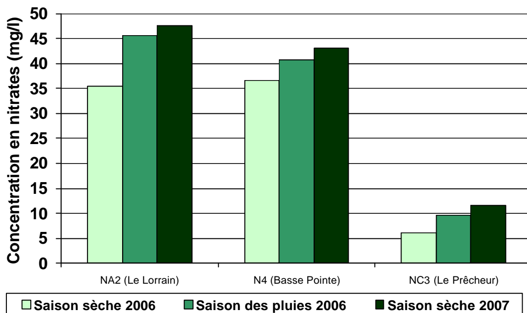
Illustration 25 : Evolution à la hausse des teneurs en nitrates sur 3 sites
