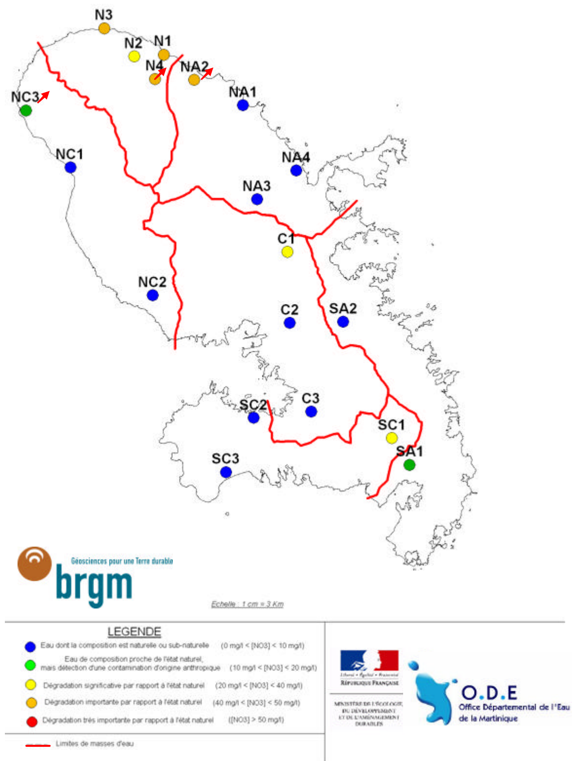
Illustration 27 : Carte des teneurs en nitrates mesurées en saison sèche 2007
