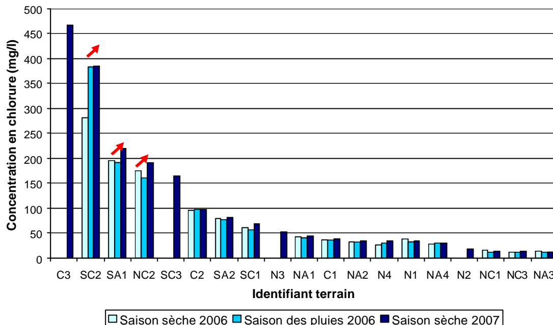
Illustration 12 : Histogramme des concentrations en chlorures mesurées en saison sèche 2007
